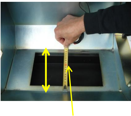
Leveyden mittaus reunasta reunaan, yli tuhka-aukon
