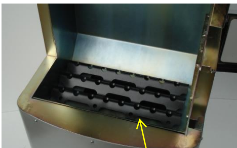
Asennettu arina kiukaan pohjalle. Nyt arina hapettaa koko pohjapinta-alan ja antaa näin hyvän palotapahtuman.
